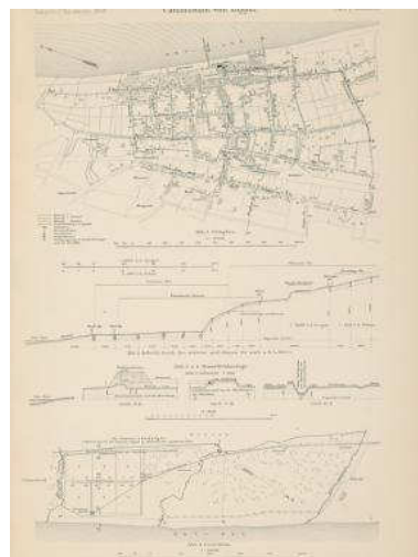
Plan Kanalizacji Sopotu. Atlas Dziennik Inżynierii Cywilnej, opublikowany przez Ministerstwo Robót Publicznych, Vol. 49, 1899.
