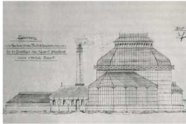
Boczny rzut projektu szklarni na terenie posiadłości Herbstów, rysunek z 1908 r. (MS Muzeum Sopotu, APG O. Gdynia)
